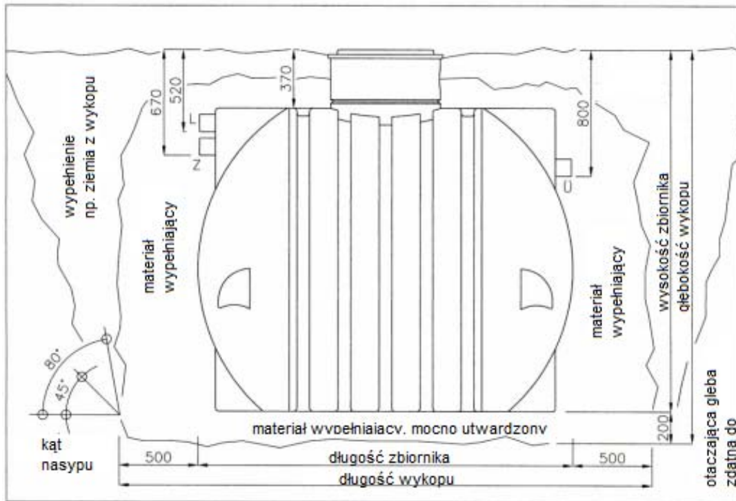
Ilustracja nr 3: Schemat i parametry zabudowy zbiornika
